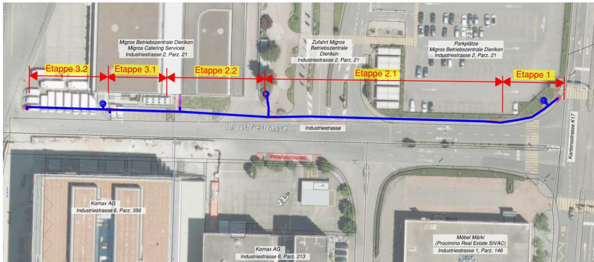
Abbildung 2: Übersicht Leitungsersatz (blau), Etappierung (rot)
