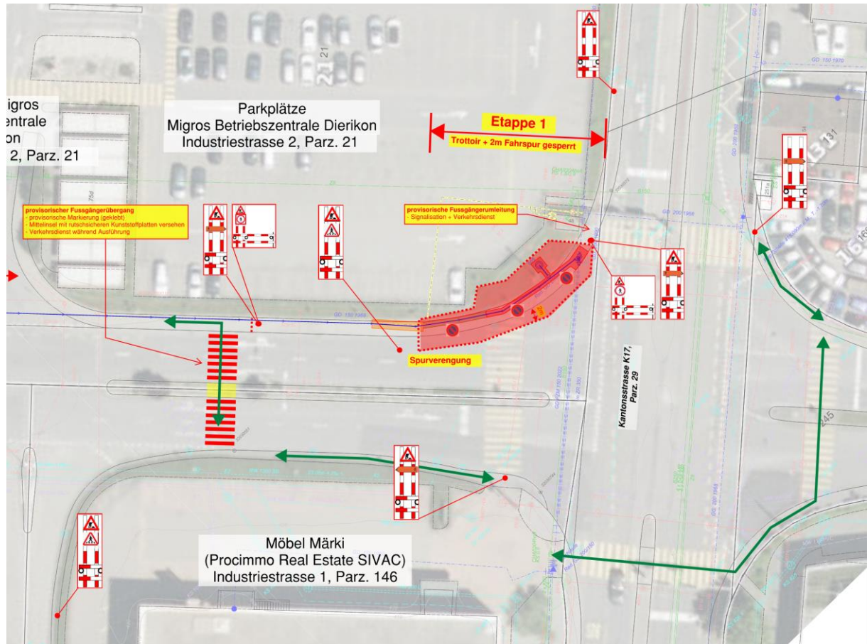
Abbildung 3: Fussgängerumleitung
